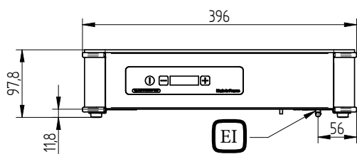
Oldalnézet
